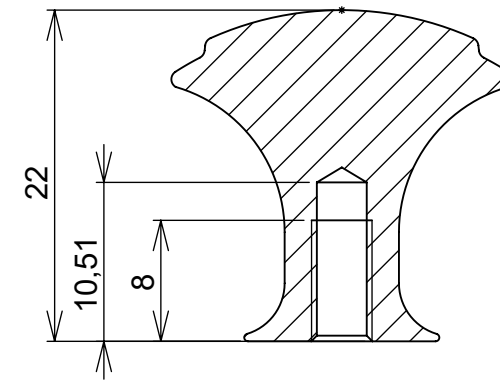
SEÇÃO F-F ESCALA 2 : 1
